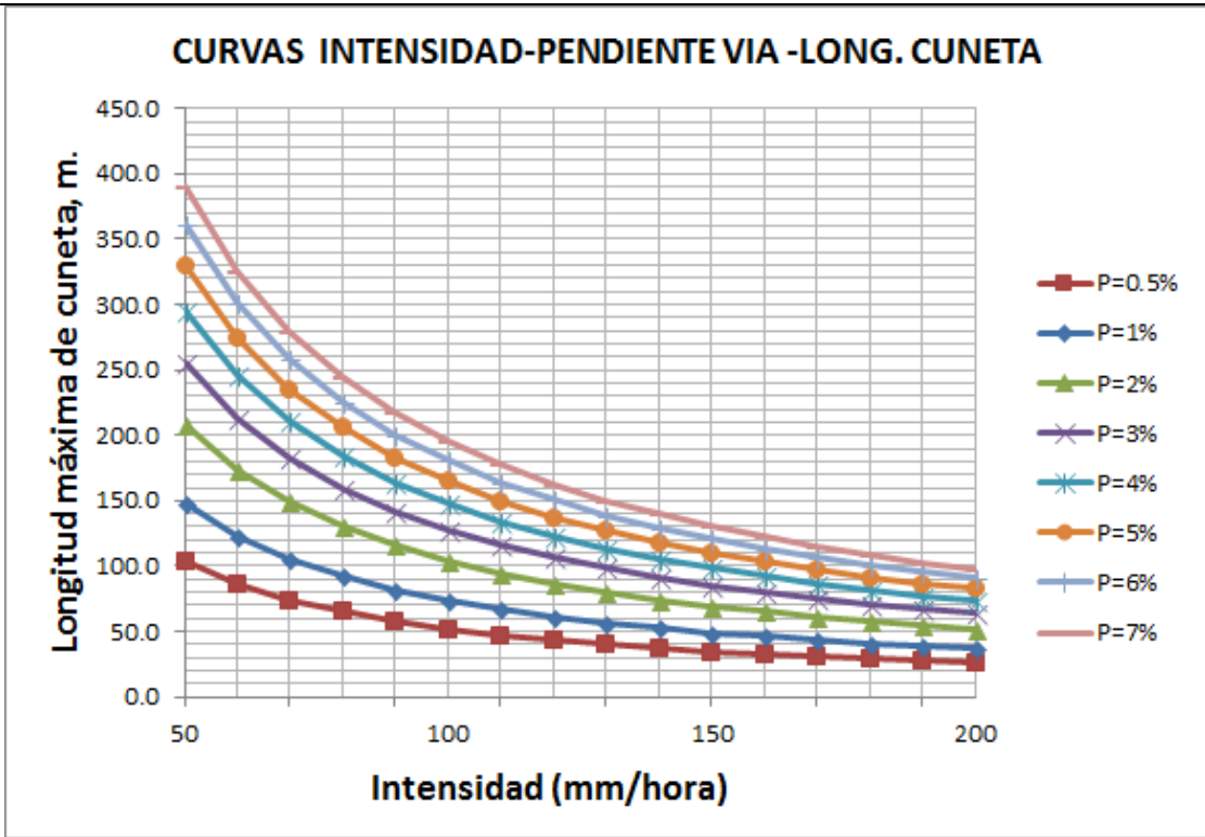
Figura 5.6 Curvas I-P-L para pendientes de vía de 0.5% a 7%
