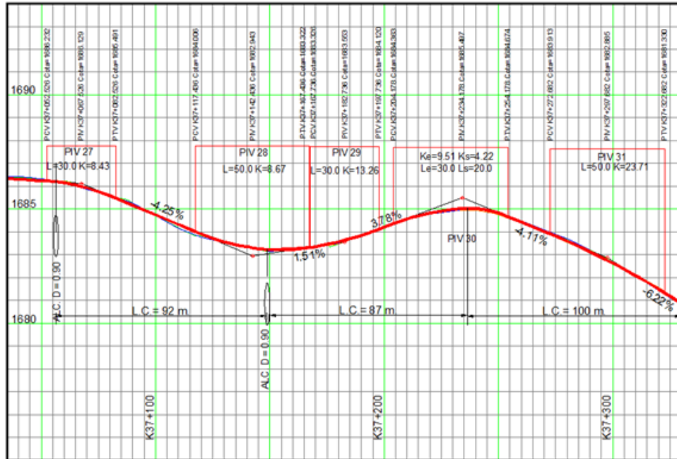
Figura 5.9 Ejemplo de localización de alcantarillas
