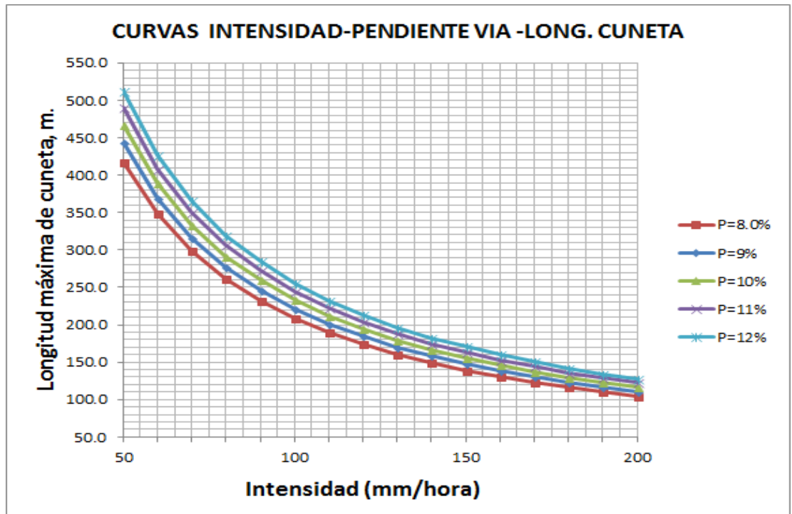
Figura 5.7 Curvas I-P-L para pendientes de vía de 8% a 12%
