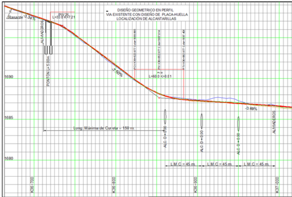
Figura 5.8 Ejemplo de localización de alcantarillas
